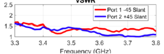
VSWR
