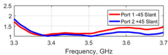
VSWR
